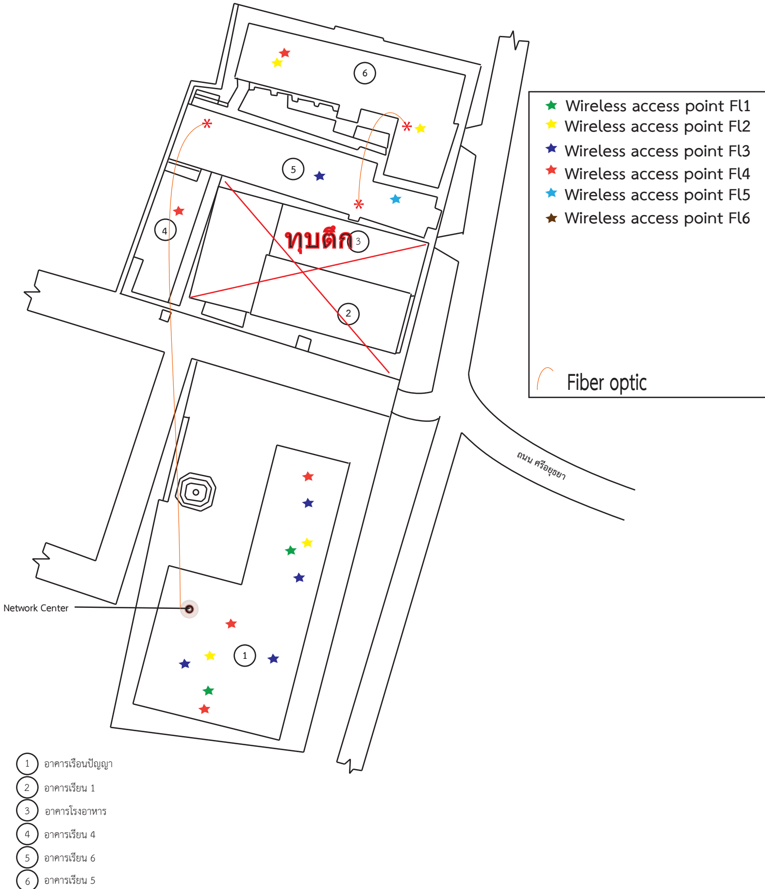
สวท.2.1-1-2 แสดงการกระจายของเส้นทางเครือข่ายชนิดมีสายและไร้สายในพื้นที่ศูนย์โชติเวช
